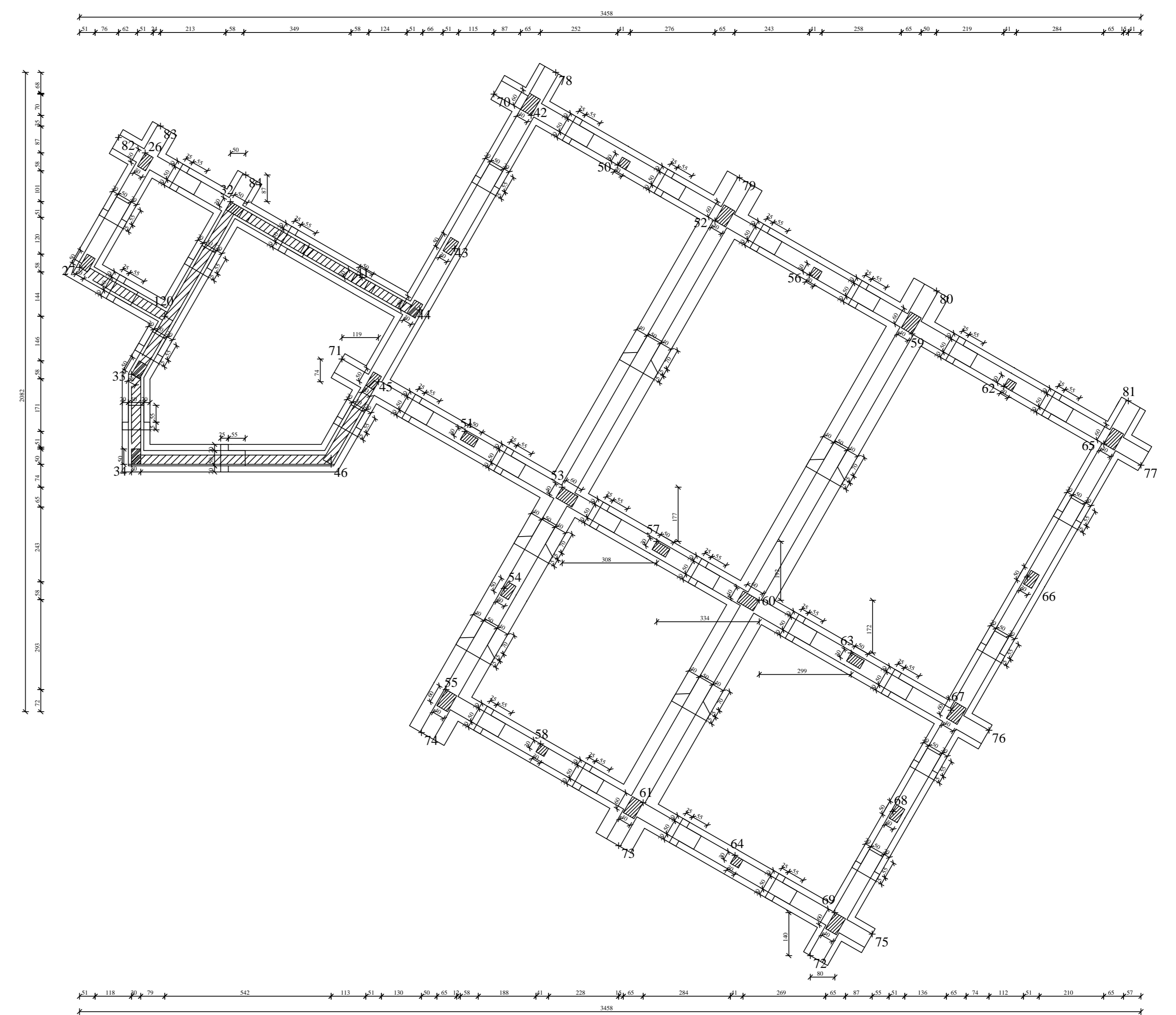
PIANTA IMPALCATO QUOTA m.-2.20 SCALA 1:100
