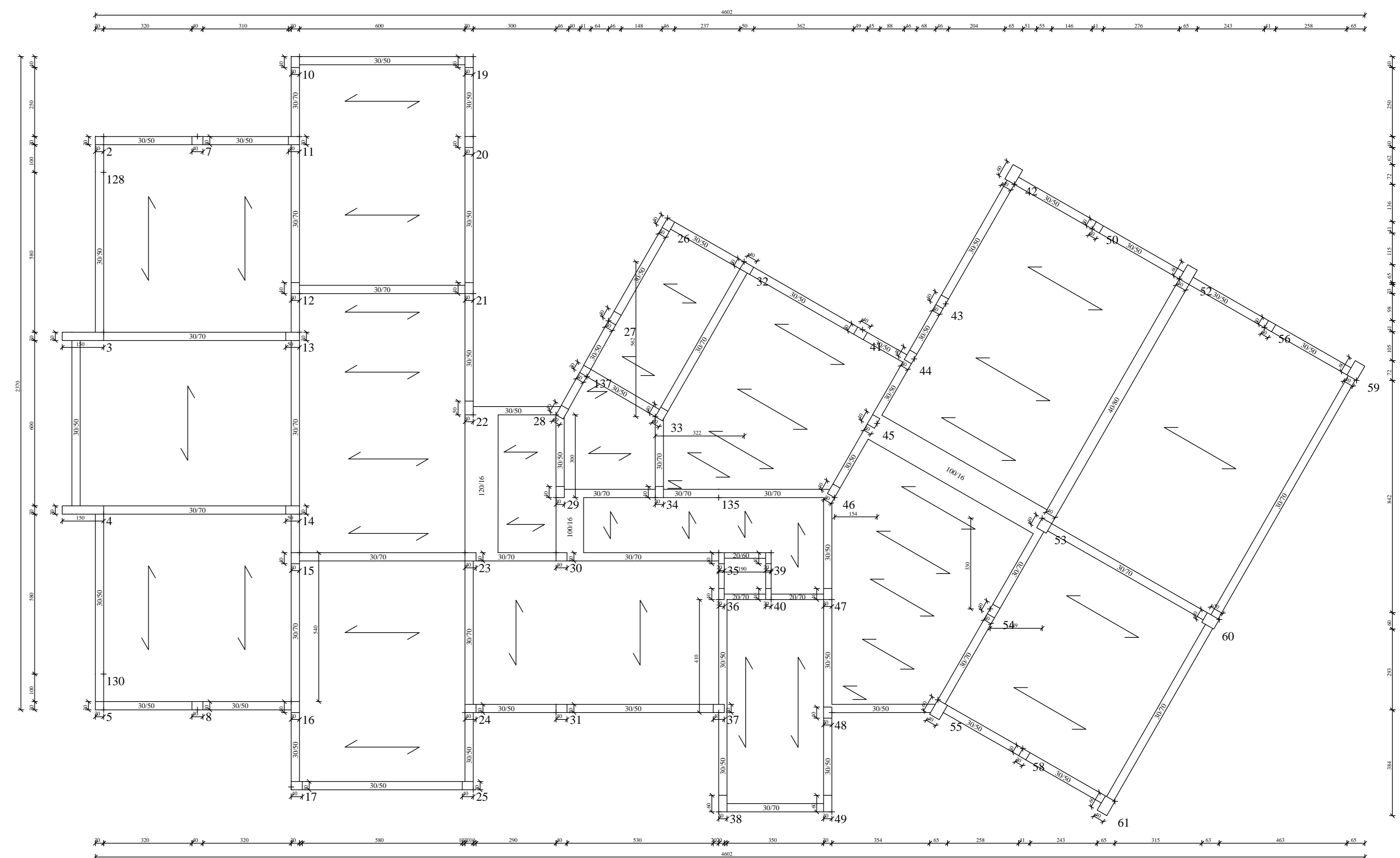
PIANTA IMPALCATO QUOTA m: 9.86 SCALA 1:100
