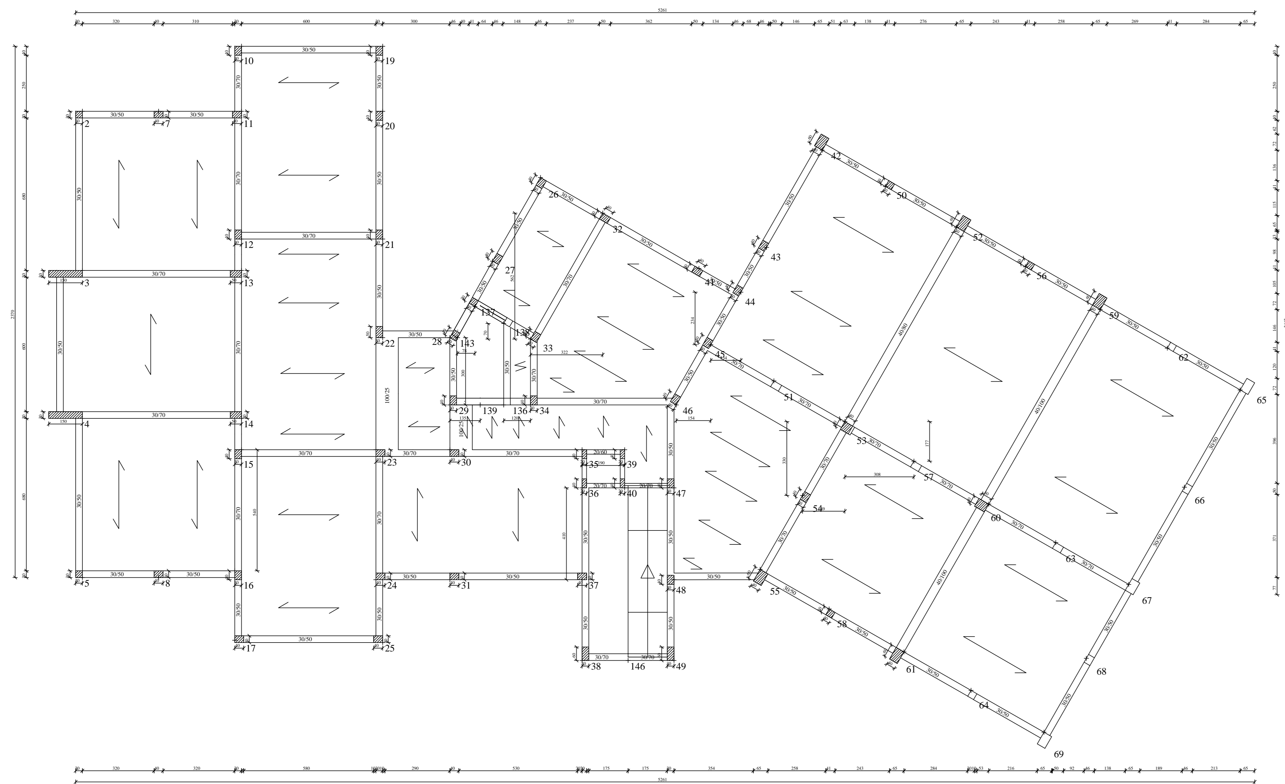
PIANTA IMPALCATO QUOTA m: 6.70 SCALA 1:100
